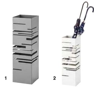
new 1. LFS-180GY 207404 2. LFS-180WH 207411 ¥3,500 (税別) W15.5×D15.5×H49cm 傘立て ロット6 (アソート可) スチール (粉体塗装)
